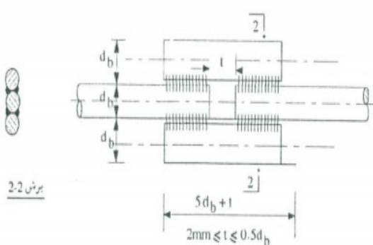
شکل (۸-۸) وصله های جوش شده از پشت و رو
