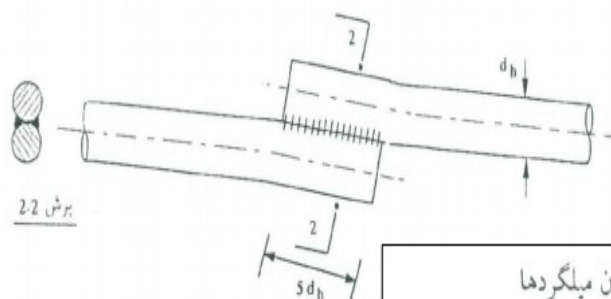
شکل (۵-۸) اتصال با نوار جوش دوطرفه
