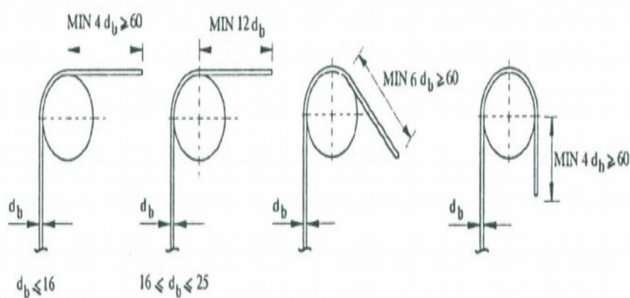
فللهای استاندارد برای میلگرد (به جز خامونها)
