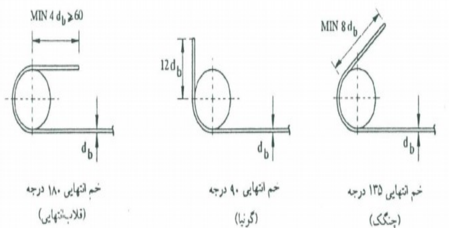
شکل شماره 2 - فللهای استاندارد
