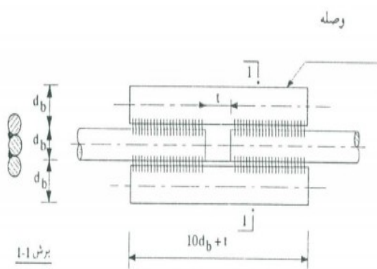
وصله های جوش شده از یک رو
