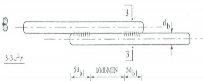
اتصال با نوار جوش بدون خم کردن میلگردها
