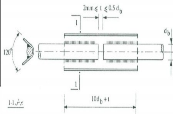
اتصال با یک وصله جانبی
